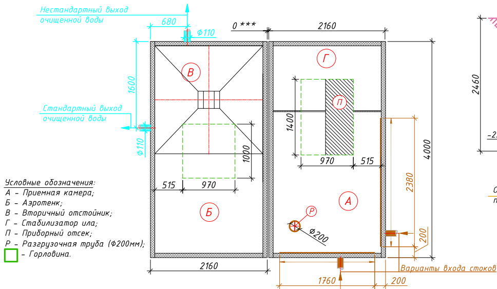
Схема станции
